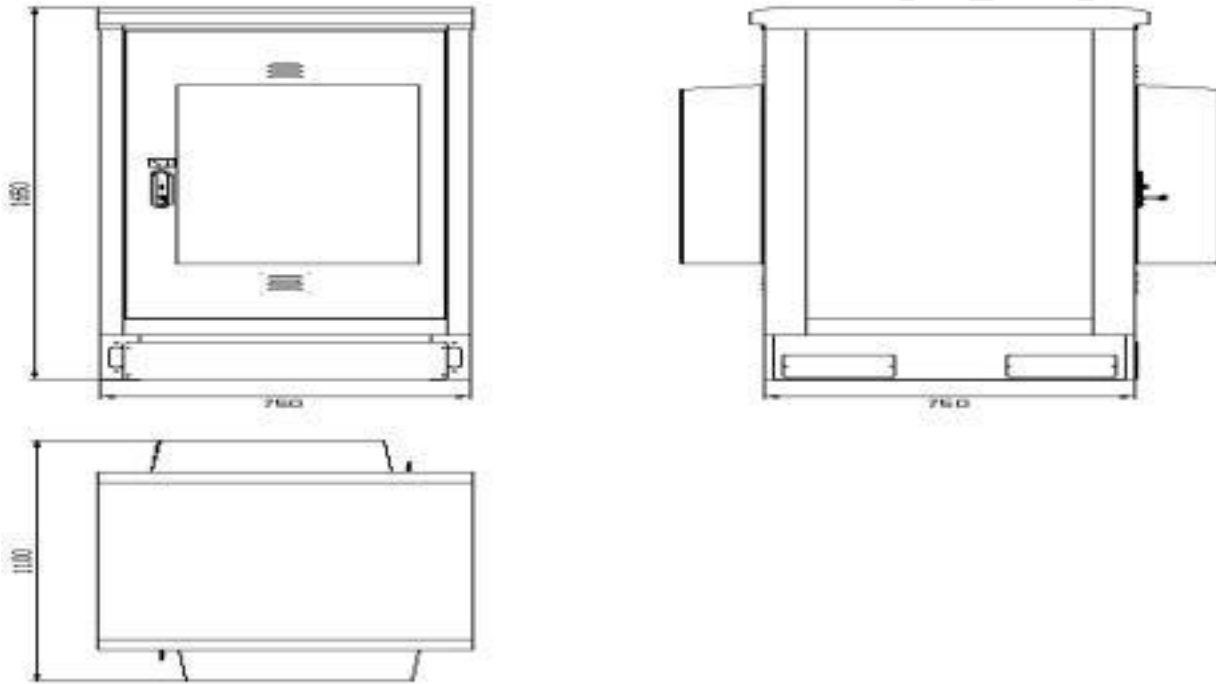
风冷型供电设备外形尺寸图
