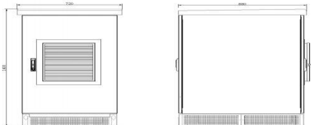
风冷型供电设备外形尺寸图
